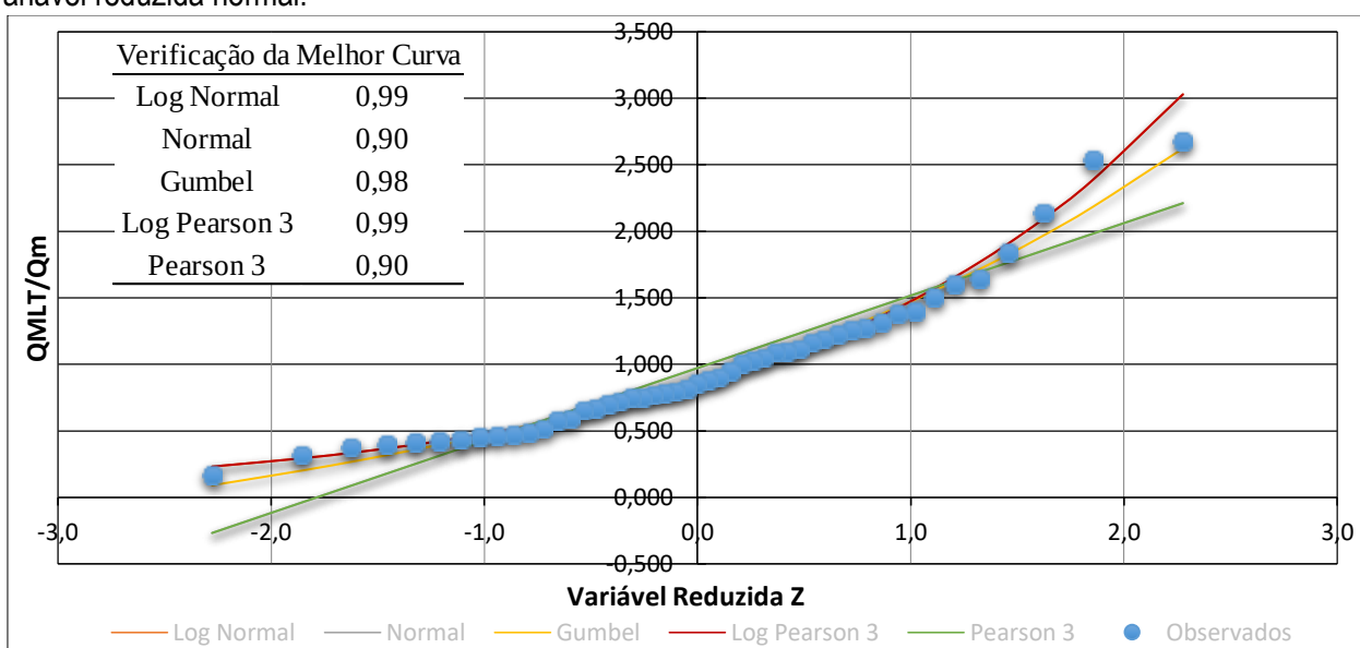
Figura 5 – Plotagem das observações adimensionalizadas pela Q_{MLT} do Baixo Itapecuru em função da variável reduzida normal.
