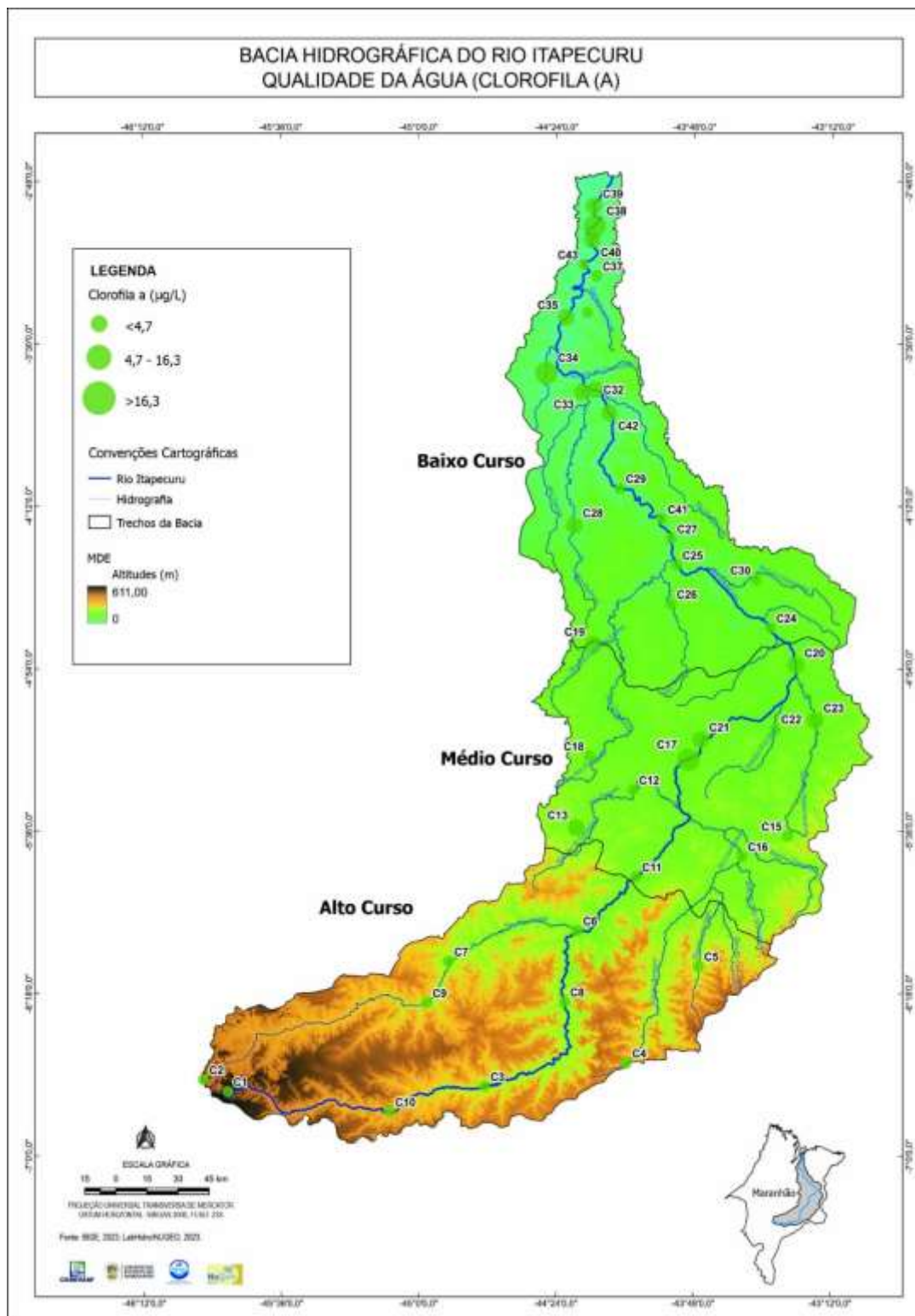
Figura 71: Clorofila-a nas águas da bacia do rio Itapecuru.
