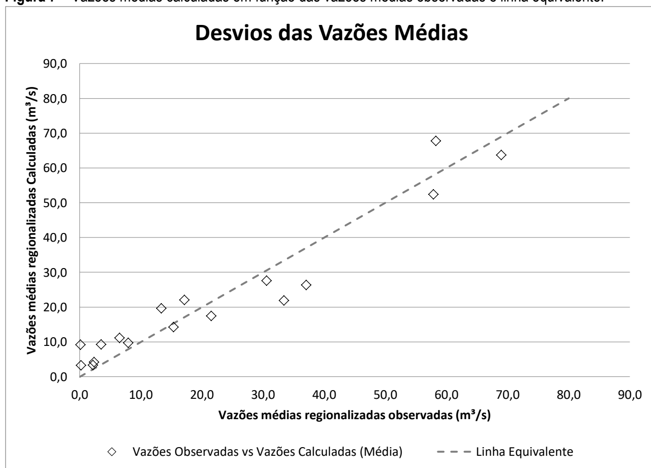
Figura 7 – Vazões médias calculadas em função das vazões médias observadas e linha equivalente.
