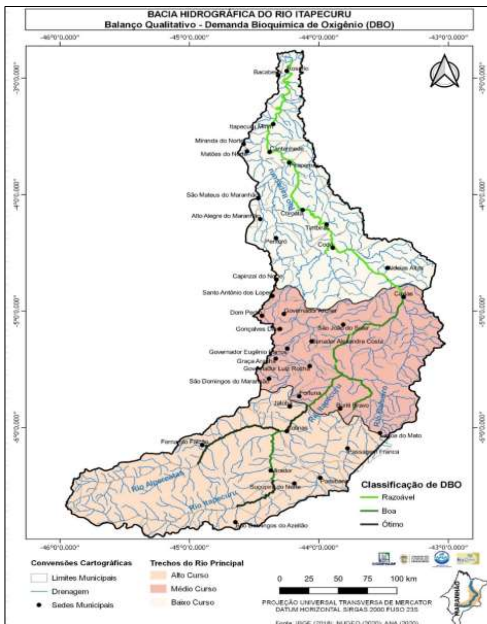
Figura 45: Balanço qualitativo da Demanda Bioquímica de Oxigênio na Bacia do rio Itapecuru.
