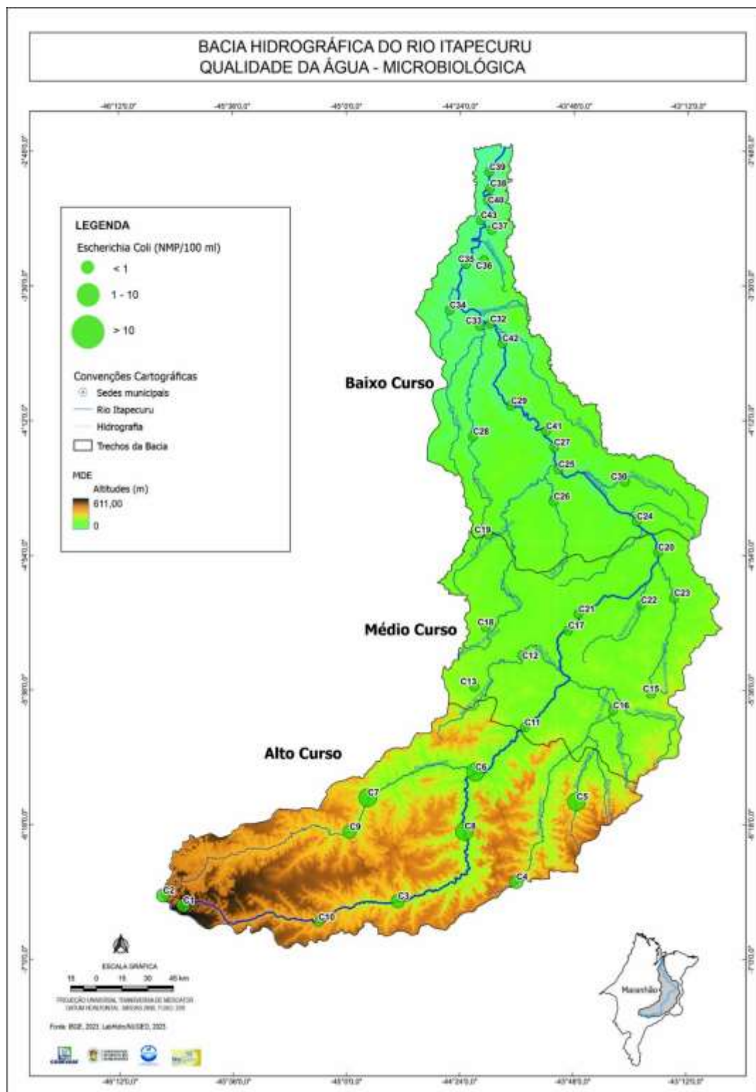
Figura 70: Escherichia coli das águas da bacia do Itapecuru.
