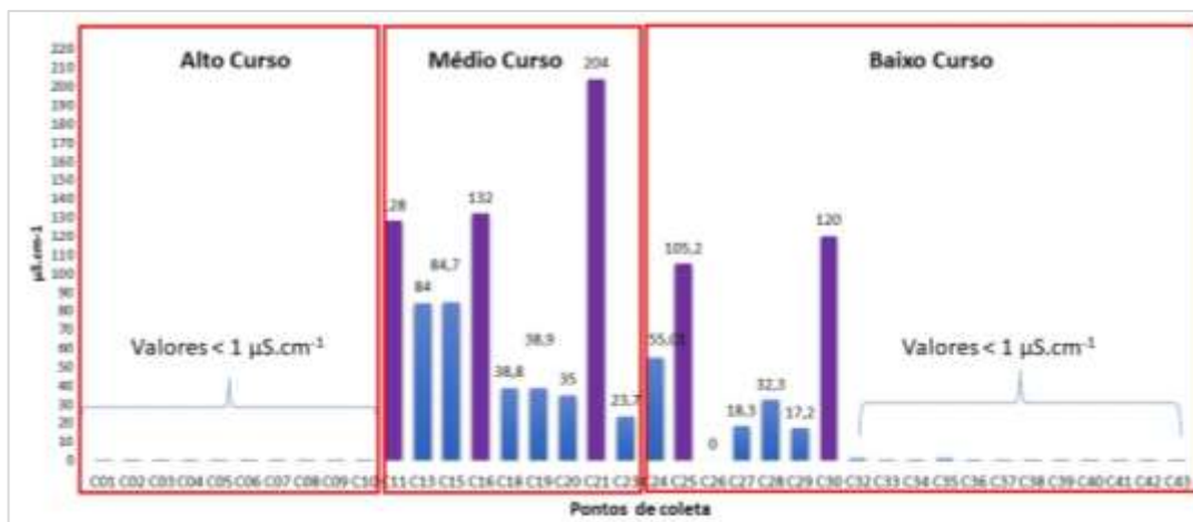
Figura 55: Condutividade elétrica das águas da bacia do rio Itapecuru.
