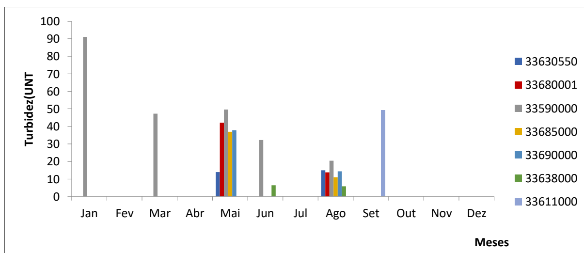
Figura 38: Comportamento da turbidez no Baixo Curso da bacia do rio Itapecuru.
