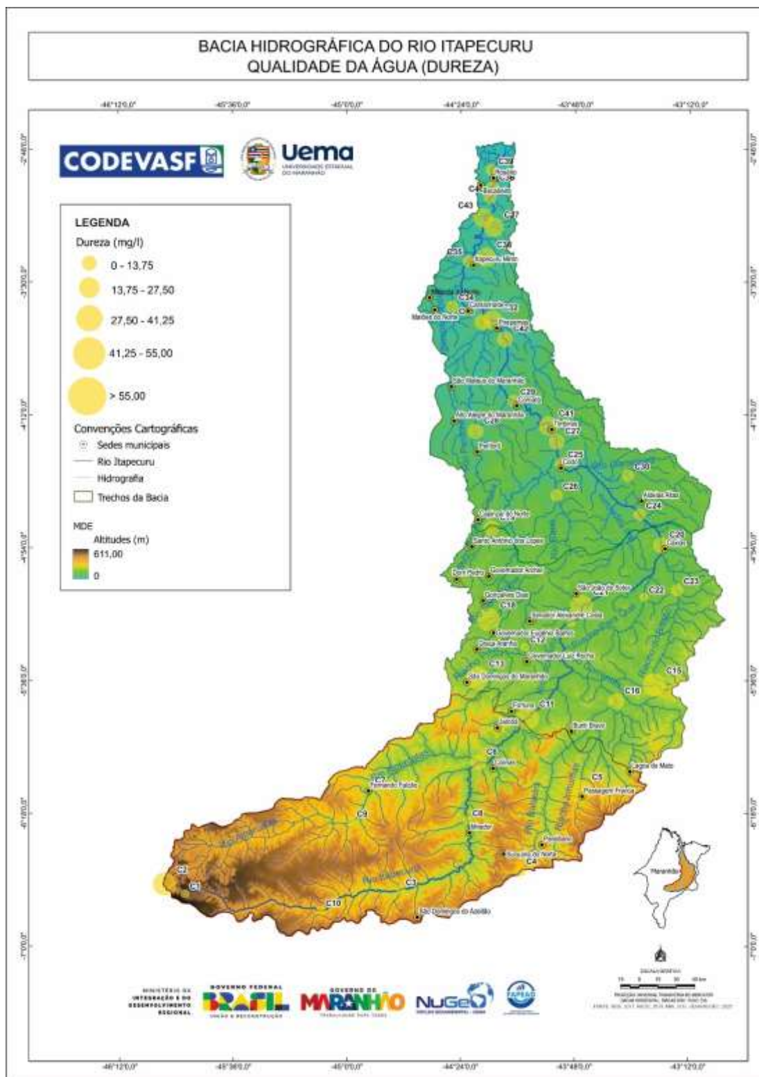
Figura 59: Dureza das águas na Bacia do rio Itapecuru.
