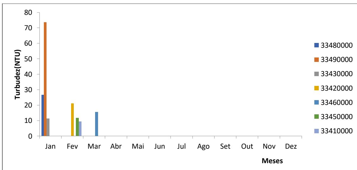
Figura 40: Comportamento da turbidez no Alto Curso da bacia do rio Itapecuru.
