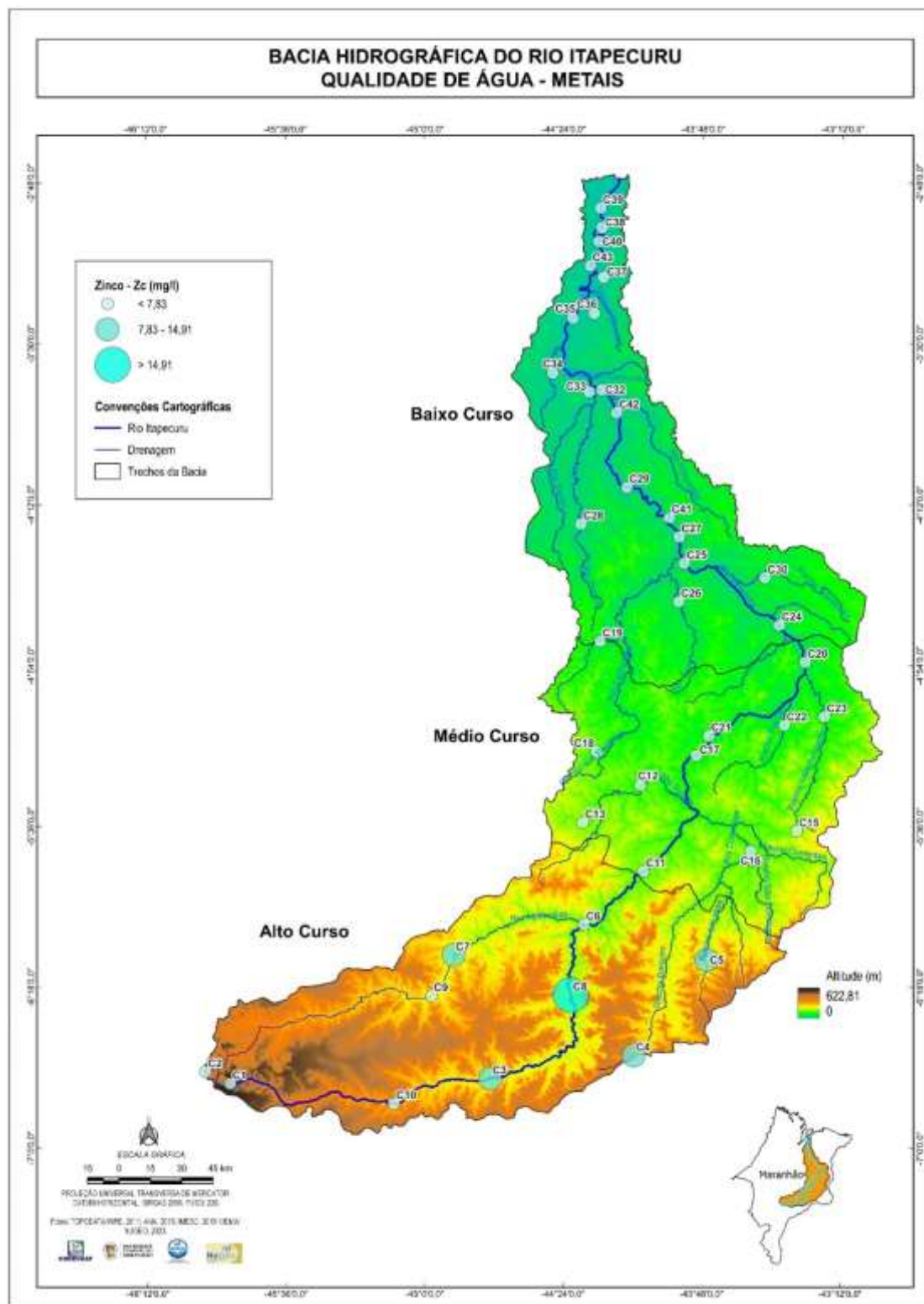
Figura 80: Zinco nas águas da bacia do rio Itapecuru.
