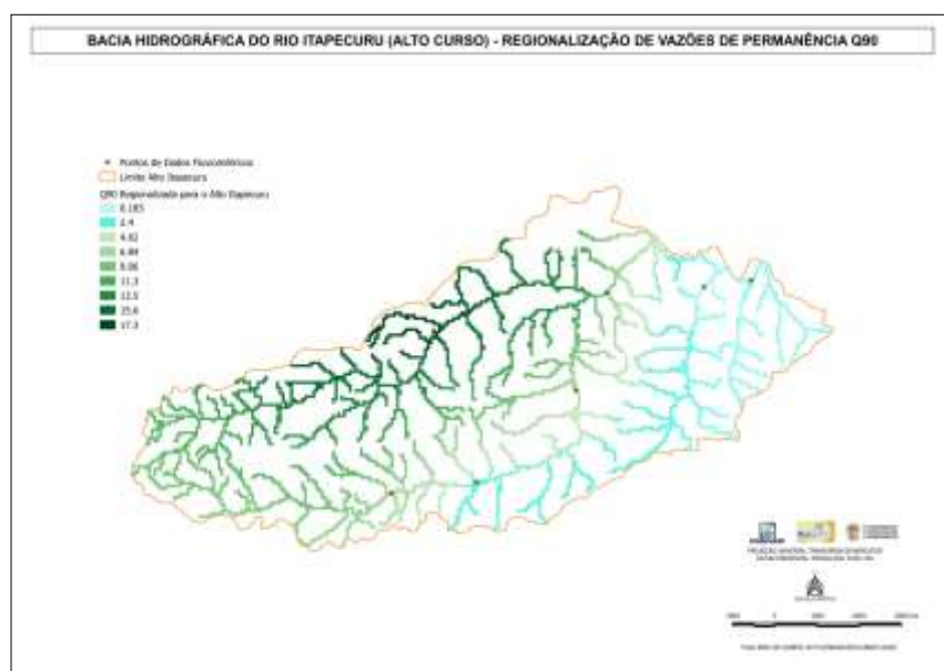
Figura 11 – Regionalização das vazões Q90 do Alto Curso do Rio Itapecuru.
