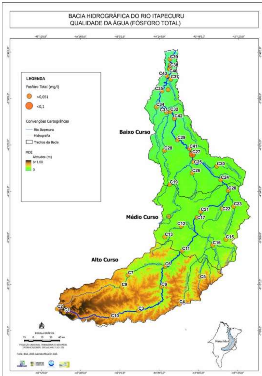
Figura 67: Fósforo das águas na Bacia do rio Itapecuru.
