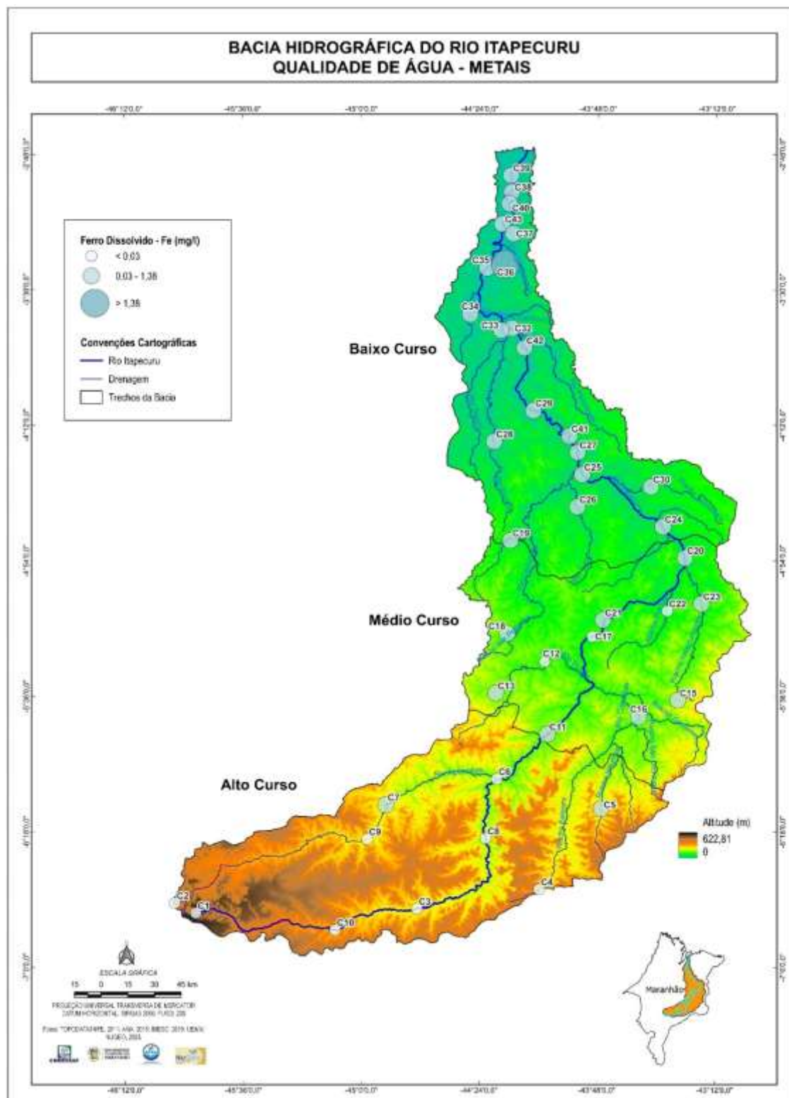
Figura 76: Ferro Dissolvido nas águas da bacia do rio Itapecuru.
