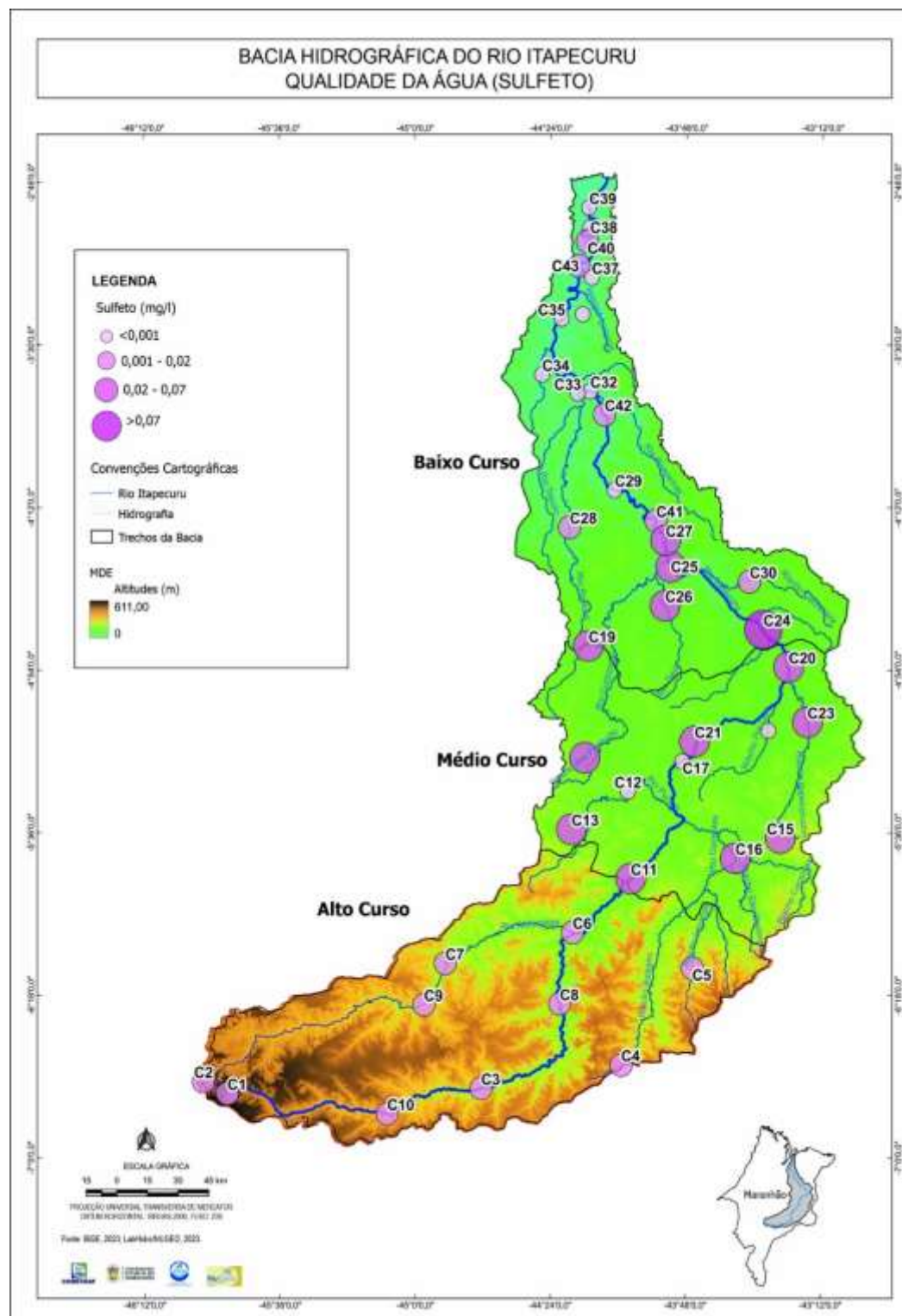
Figura 63: Sulfeto das águas na Bacia do rio Itapecuru.
